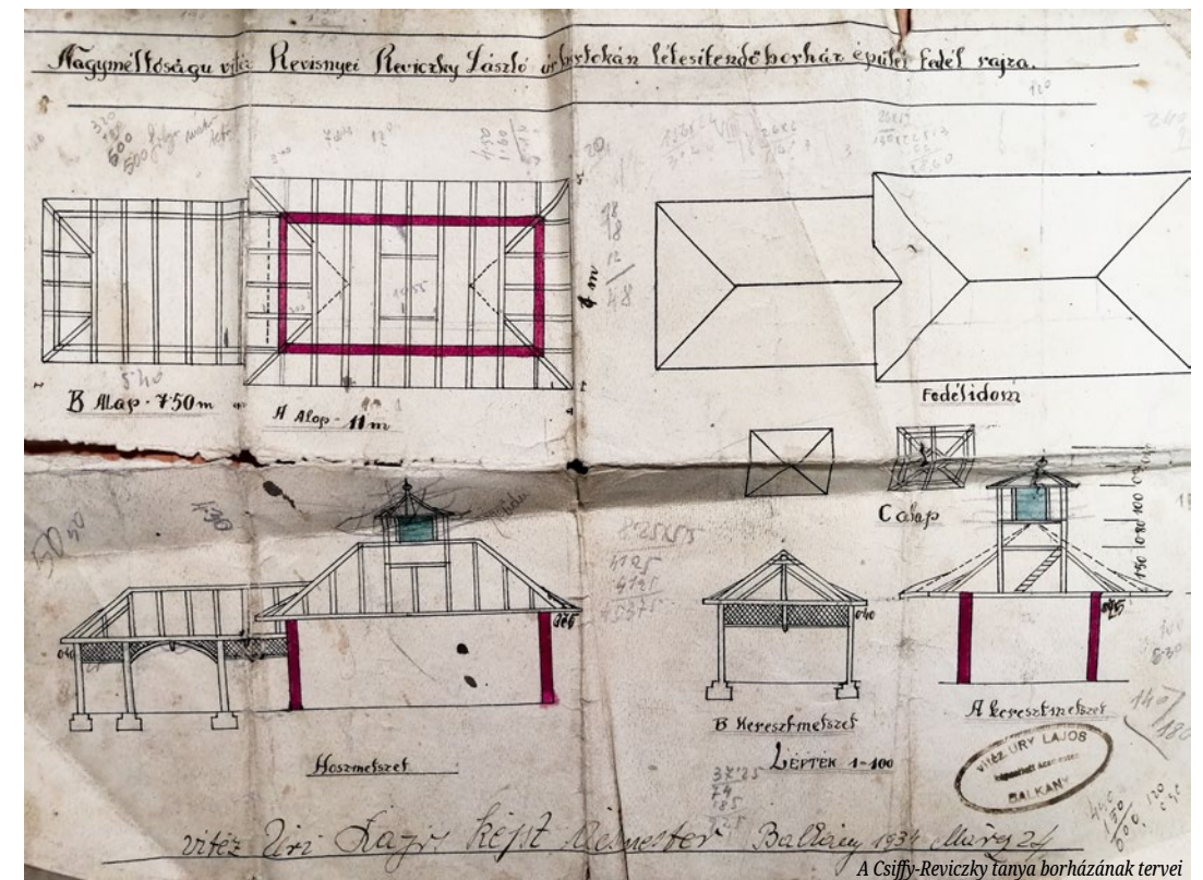
A Csiffy-Reviczky tanya borházának tervei
